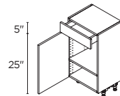
1 DOOR / 1 DRAWER 15" | B1514(L/R) 18" | B1814(L/R) 24" | B2414(L/R)
